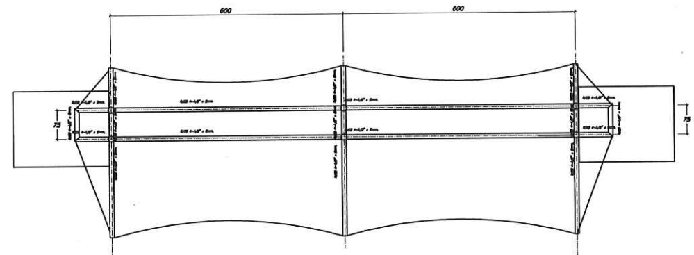
PLANTA DE ESTRUCTURACION DE CUBIERTA MODULO "A". EBO. 1.00
