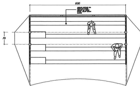
PLANTA ARQUITECTONICA DE GRADERIA MODULO "B". EBO. 1/25
