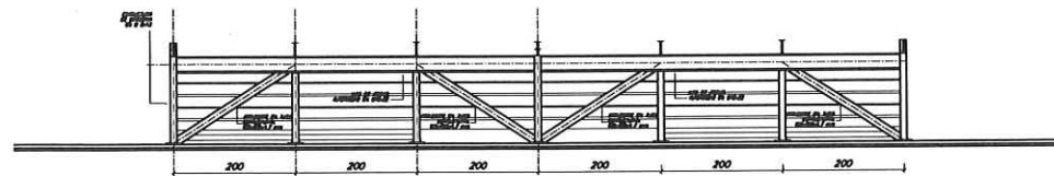
ELEVACION LONGITUDINAL POSTERIOR DE MODULO DE GRADERIA TIPO "B". EBO. 1.00
