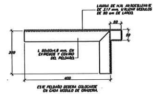
DETALLE DE PELDAÑO DE EVACUACIÓN. ESC. 1:5
