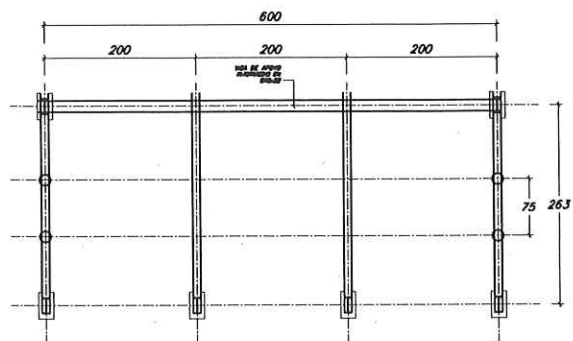
PLANTA DE ESTRUCTURACION DE GRADERIA MODULO "B". EBO. 1:25
