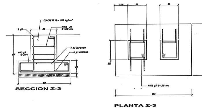
DETALLE DE ZAPATA Z-3 EBC. 1:10
