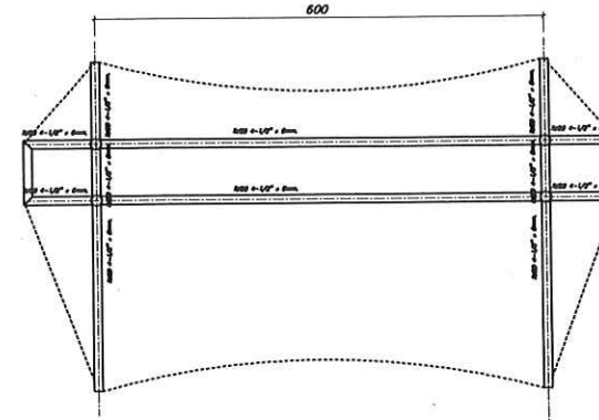
PLANTA DE ESTRUCTURACION DE CUBIERTA MODULO "B". EBO. 1/25
