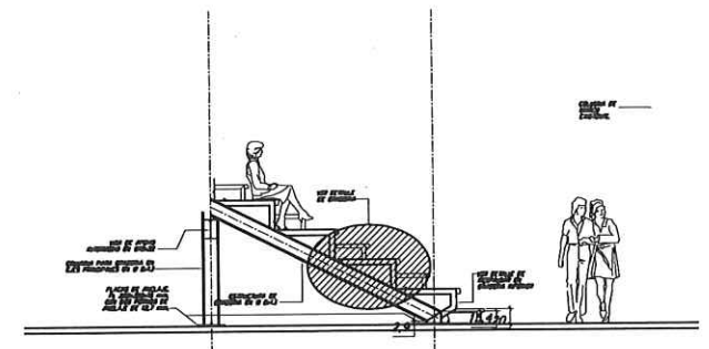
SECCION TRANSVERSAL DE MODULO DE GRADERIA. EBO. 1/25
