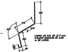
DETALLE DE RESPALDO EN GRADERIA INFERIOR. EBO. 1:5
