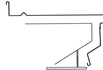
DETALLE DE RESPALDO EN GRADERIA INFERIOR. EBO. 1:5
