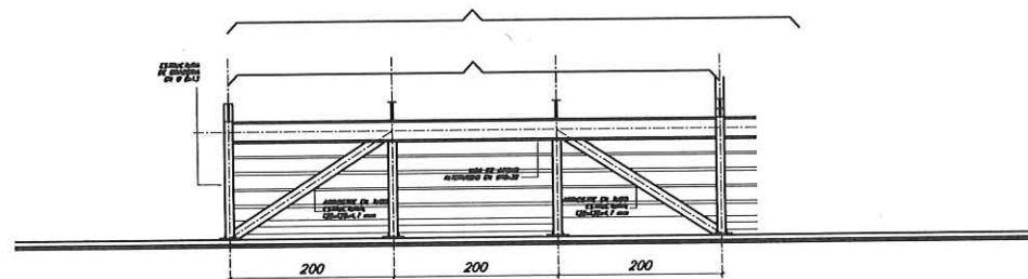
ELEVACION LONGITUDINAL POSTERIOR DE MODULO DE GRADERIA TIPO "A". EBO. 1:25
