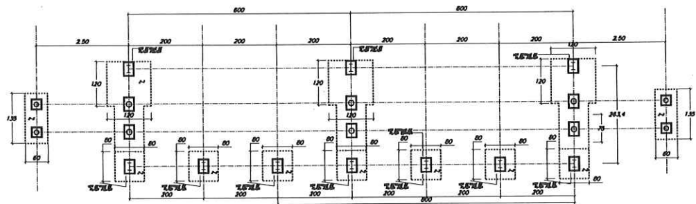
PLANTA DE FUNDACIONES PARA MODULO "A" DE GRADERIA. EMB. 1:200
