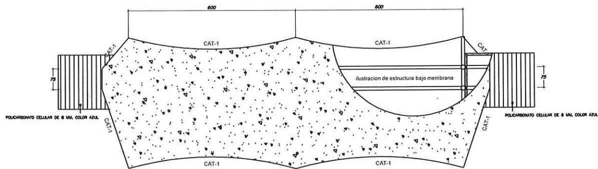
PLANTA DE MEMBRANA TENSADA DE CUBIERTA MODULO "A". EBO. 1.00
