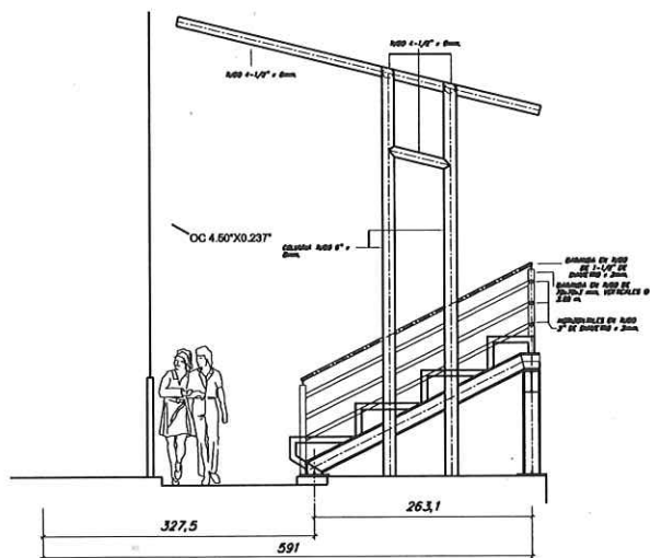
SECCION TRANSVERSAL BARANDAL DE MODULO "A" Y "B" DE GRADERIA. EBO. 1:25
