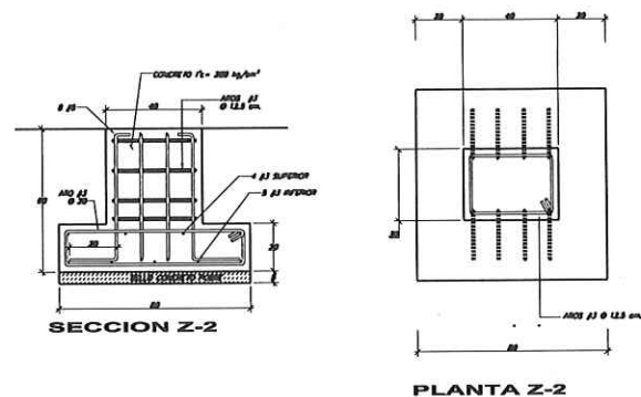
DETALLE DE ZAPATA Z-2 EBC. 1:10
