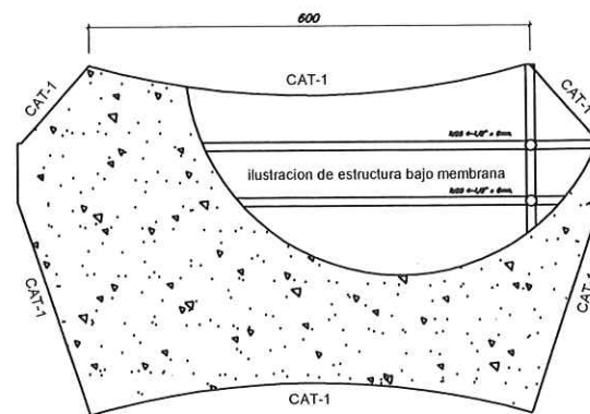
PLANTA DE MEMBRANA TENSADA DE CUBIERTA MODULO "B". EBO. 1/25
