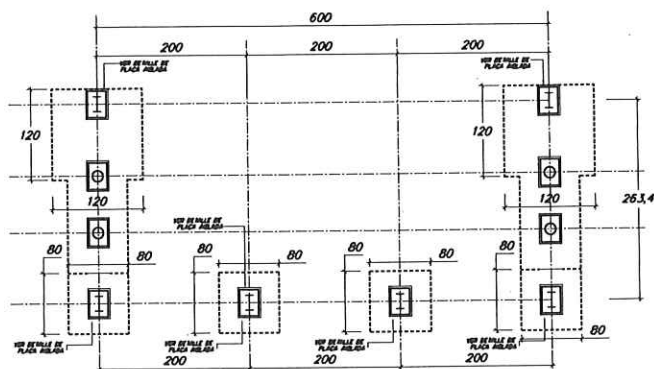
PLANTA DE FUNDACIONES PARA MODULO DE GRADERIA. EBO. 1:25
