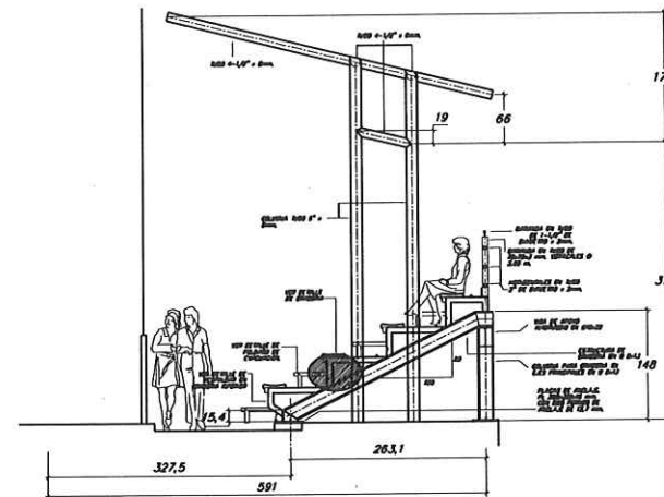
SECCION TRANSVERSAL "A" CON ANEXO PARA SILLA DE RUEDAS DE MODULO DE GRADERIA. EBO. 1/25
