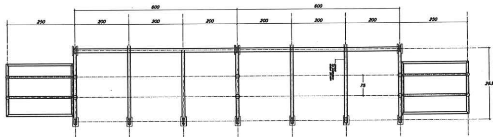
PLANTA DE ESTRUCTURACION DE GRADERIA MODULO "A". EMB. 1:200
