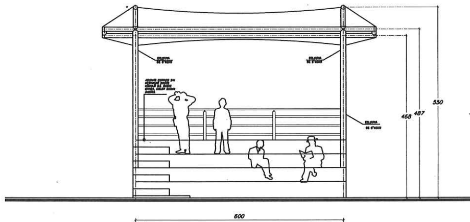
FACHADA FRONTAL DE MODULO "B" DE GRADERIA. EBO. 1/25
