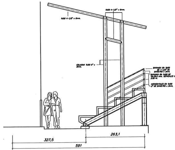
SECCION TRANSVERSAL BARANDAL INTERMEDIO DEL MODULO "A" DE GRADERIA. EBO. 1:25
